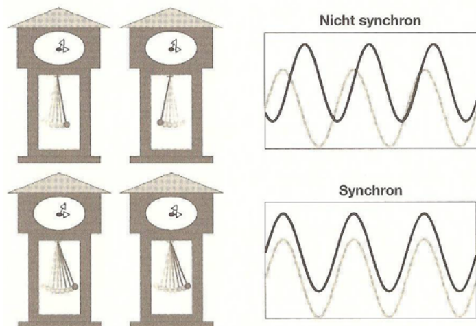
Abbildung 2.6: Harmonie (auch Entrainment; Frequenzkopplung): Wenn zwei Pendeluhren nebeneinander an einer Wand stehen, schwingen ihre Pendel im Laufe der Zeit synchron. Die Uhren erzeugen dann Wellenmuster, wie rechts unten abgebildet. Dieses Muster ist ein klassisches Beispiel für das Phänomen der Frequenzkopplung (Harmonie), das überall in der Natur (sowohl in lebenden Organismen wie auch in unbelebten Systemen) vorkommt. Allgemein lässt sich feststellen: Wenn Systeme synchronisiert sind, arbeiten sie effizienter. Im menschlichen Körper ist das Herz als der stärkste rhythmische Oszillator das zentrale „Pendel“, das den anderen Körpersystemen den „Takt“ angibt.
